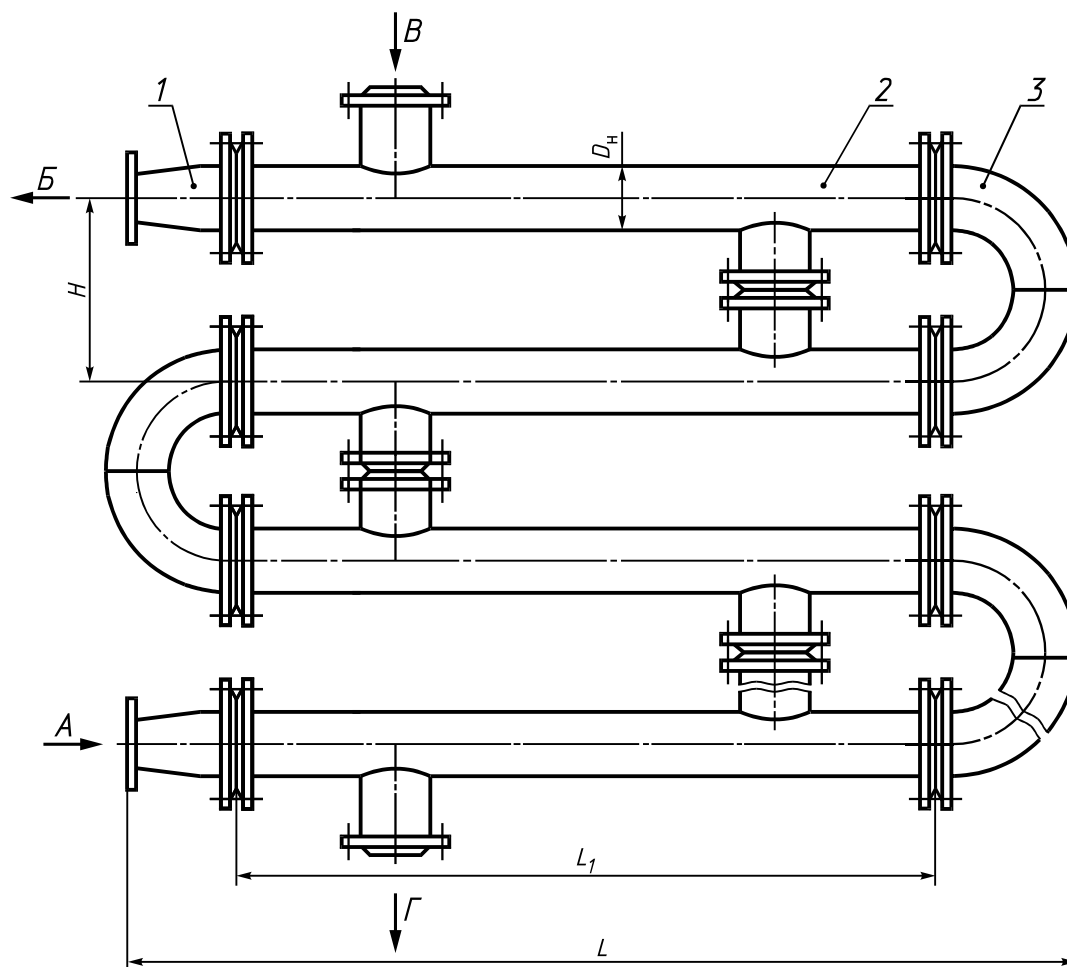
1 — переход исполнения 1 (см. рисунок 11); 2 — блок-секция типа ПБ1; 3 — калач соединительный исполнения 1 (см. рисунок 10); А — вход нагреваемой воды; Б — выход нагреваемой воды; В — вход греющей воды, Г — выход греющей воды
