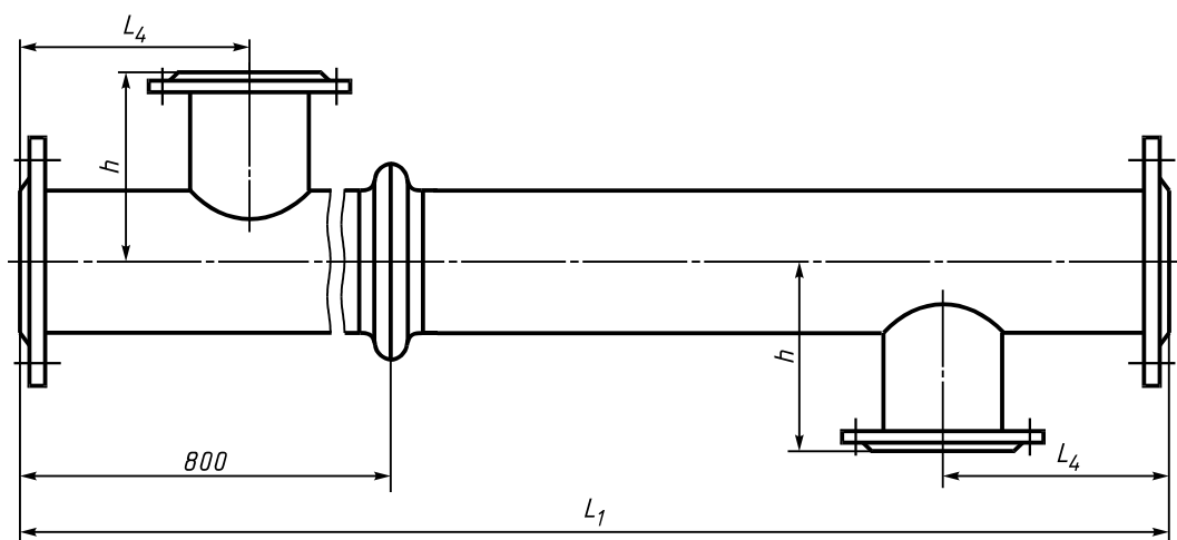
Рисунок 6 — Блок-секция типа PB1K с компенсатором и с типовым расположением патрубков
