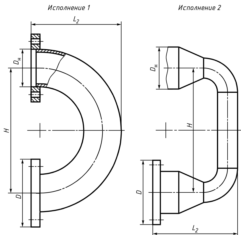
Рисунок 10 — Калач соединительный
